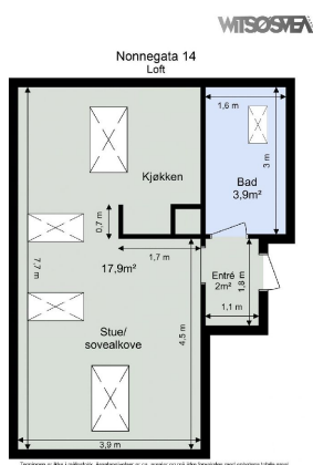
Plantegning - Leiligheten varmes opp med elektrisitet
