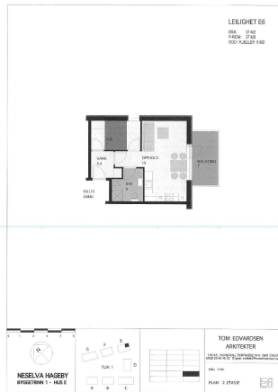
Plantegning
