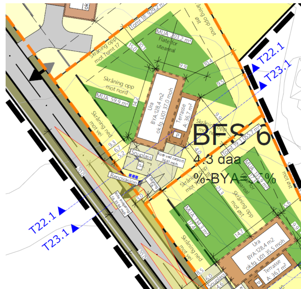
Situasjonsplan som viser sikttrekant.
