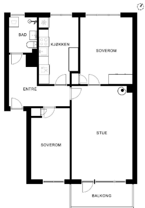
Plantegning
