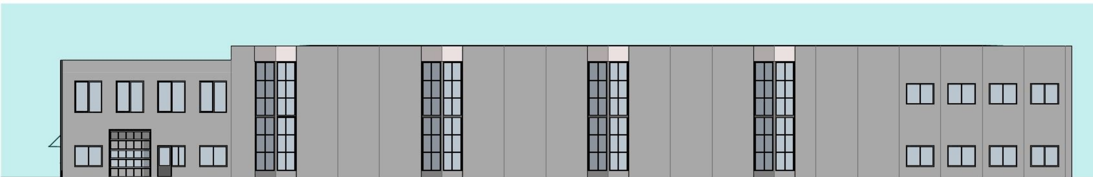
1:200 Fasade Sør
