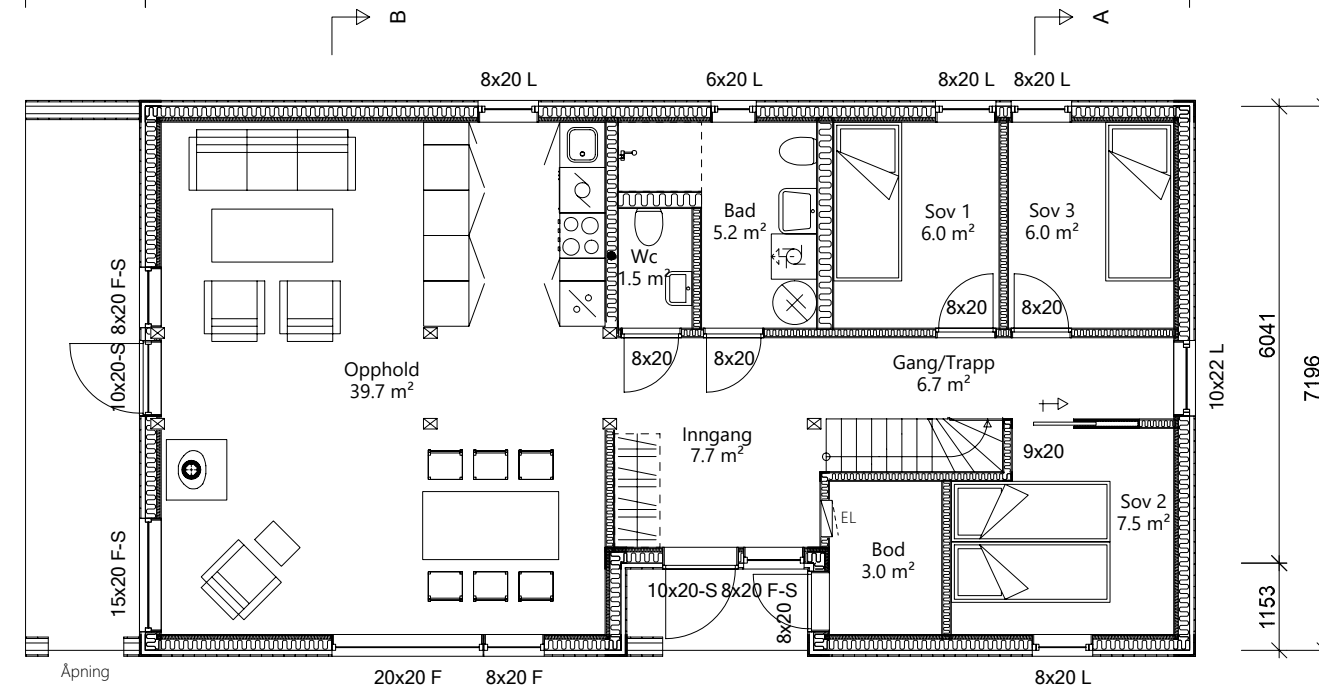
PLAN 1.ETG 1584 6292 2548 4974 15398 A B
