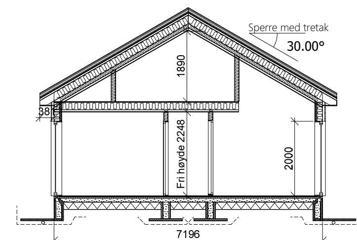
SNITT A-A
