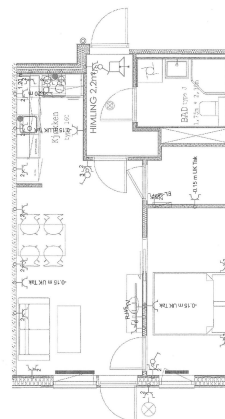
Plantegning
