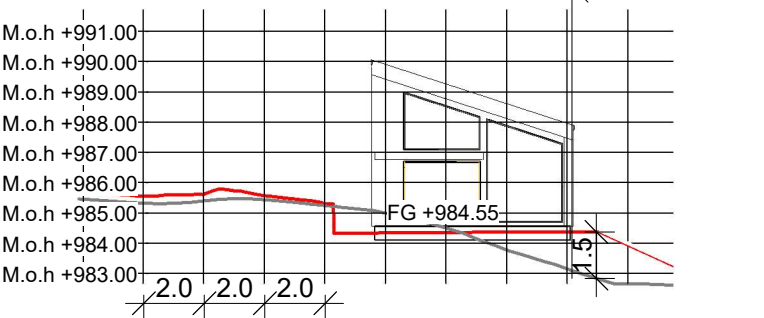
376.5_Snitt1 1 : 250
