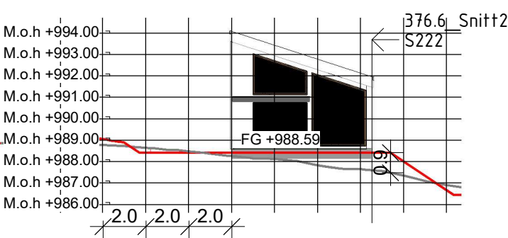
376.6_Snitt1 1 : 250
