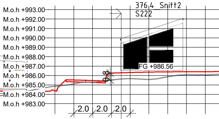
376.4_Snitt1 1 : 250
