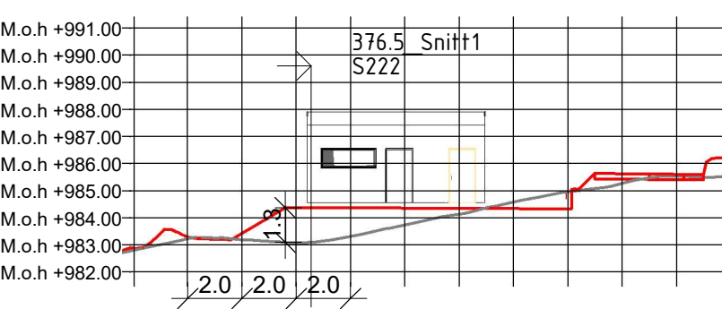
376.5_Snitt2 1 : 250
