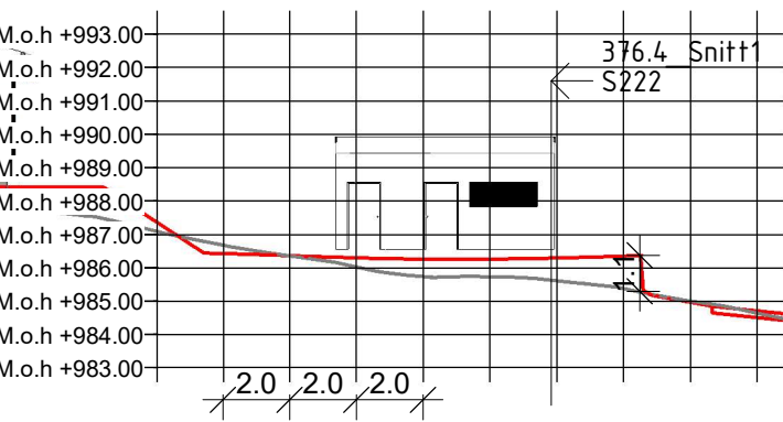
376.4_Snitt2 1 : 250
