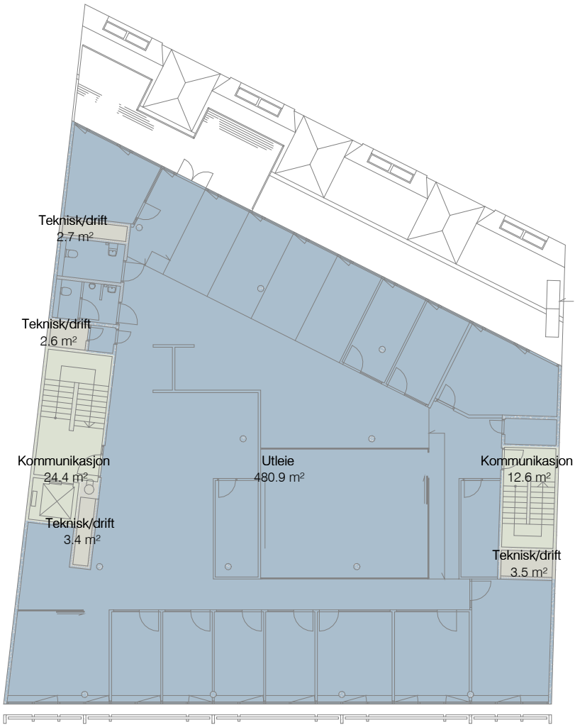
plan 04 1 : 250
