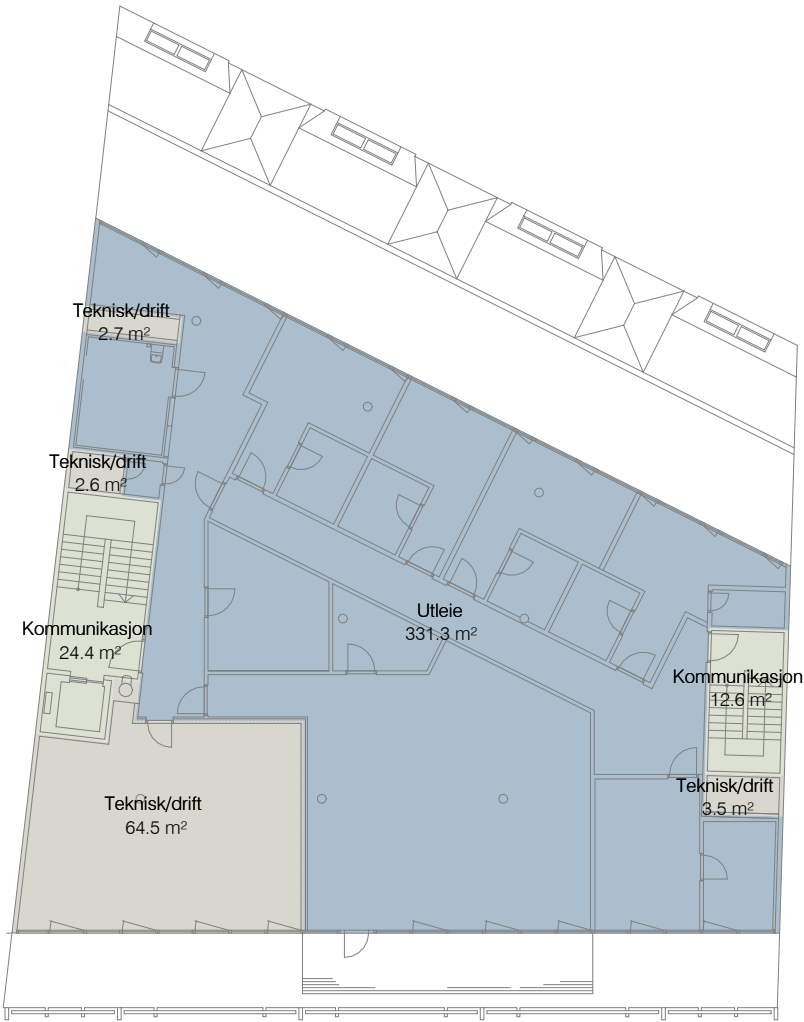
plan 06 1 : 250
