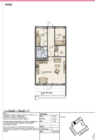
Plantegning H102
