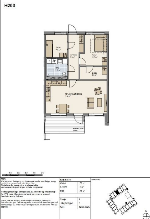
Plantegning H203
