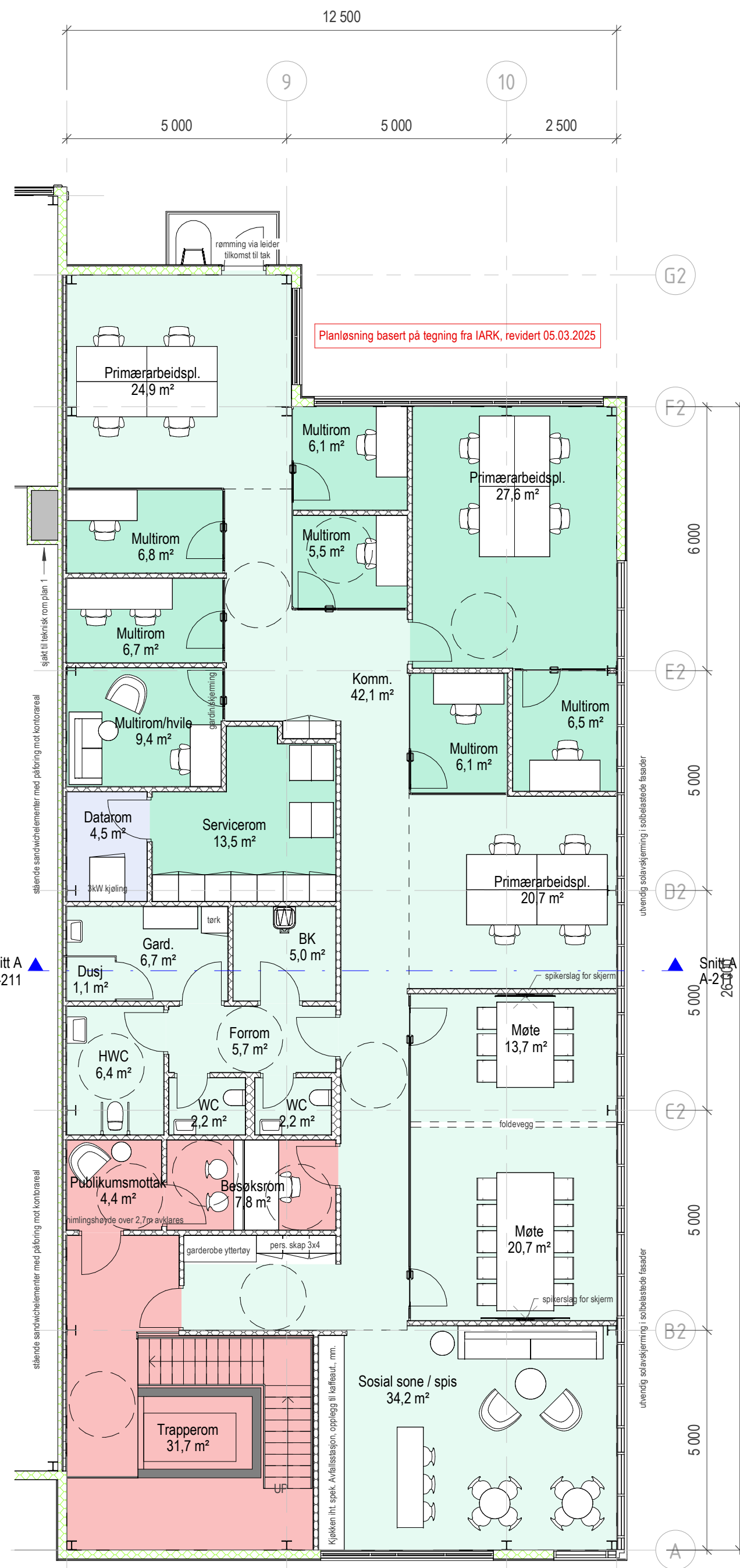
200 Plan 2 - kontor 1 : 100
