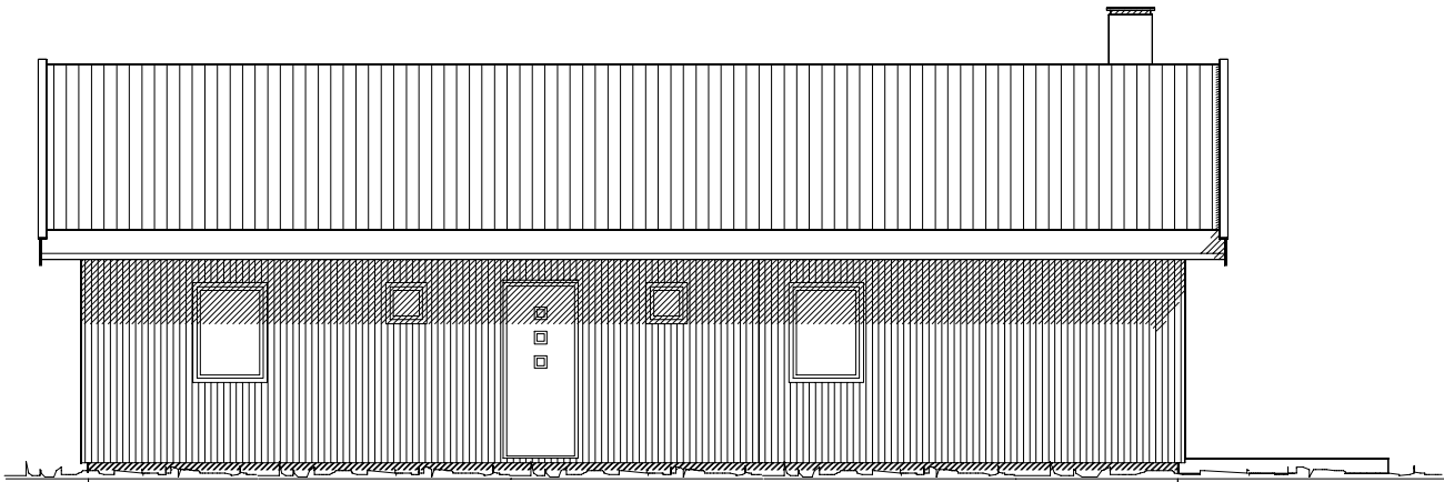
FASADE 3
