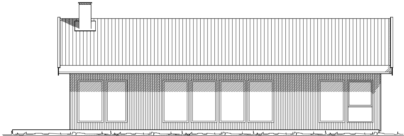
FASADE 1
