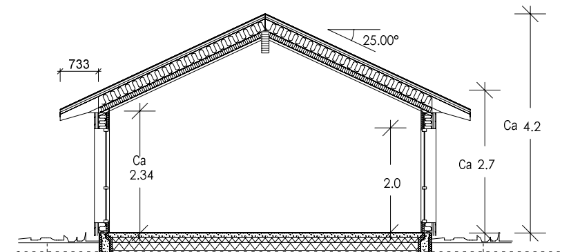
SNITT B - B
