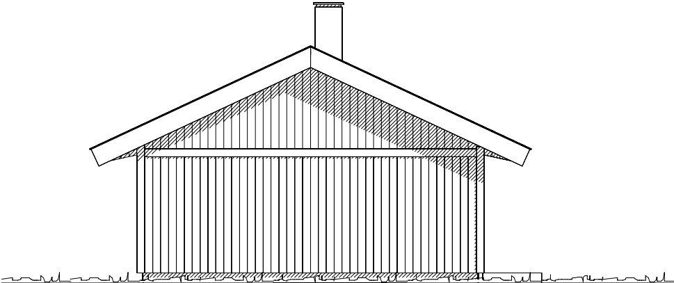
FASADE 4
