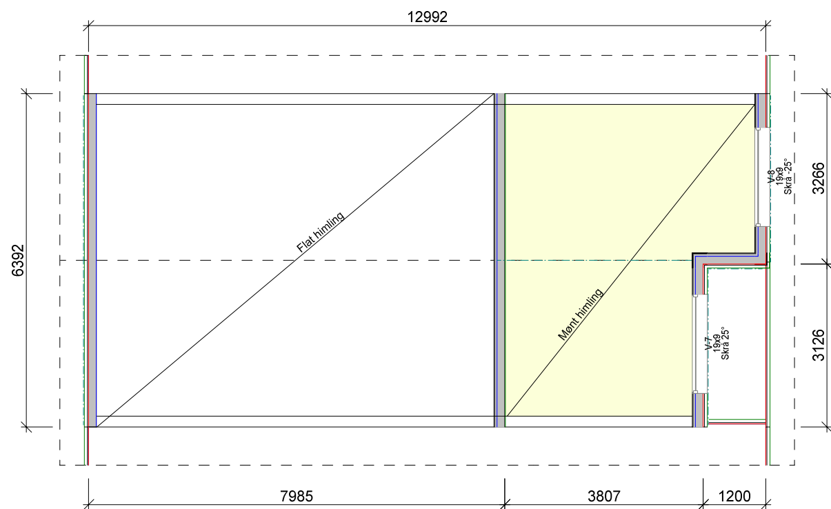
PLAN TAK
