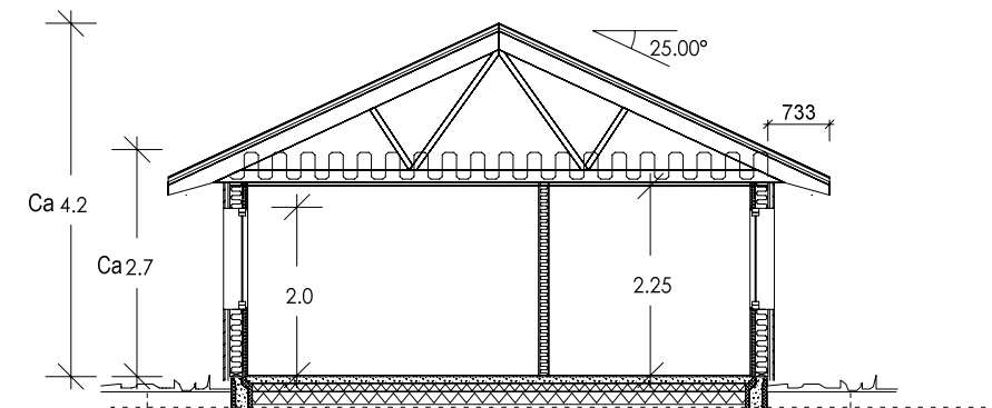
SNITT A - A
