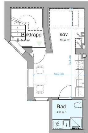
Plantegning
