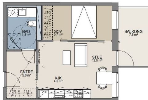
Plantegning
