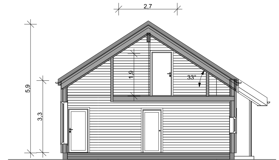
7.8 SNITT A-A
