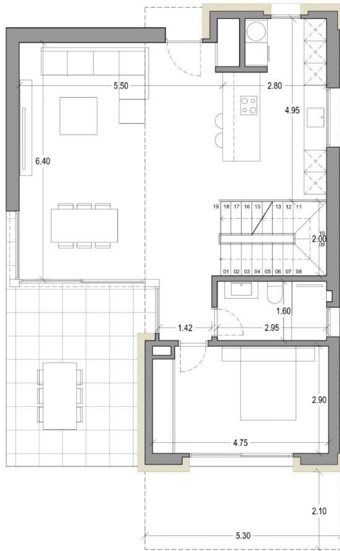
PLANTA BAJA - COTAS
