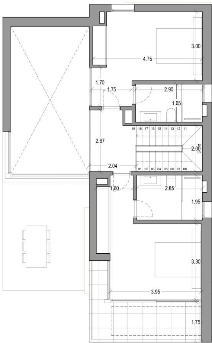
PLANTA ALTA - COTAS
