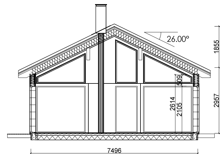
Snitt B-B
