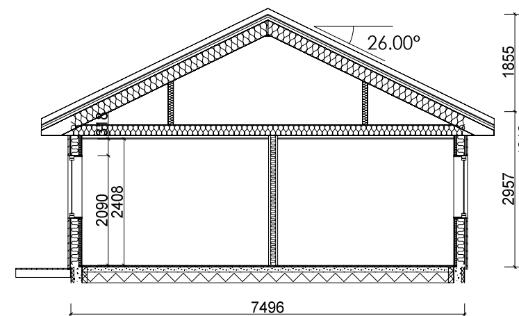
Snitt A-A
