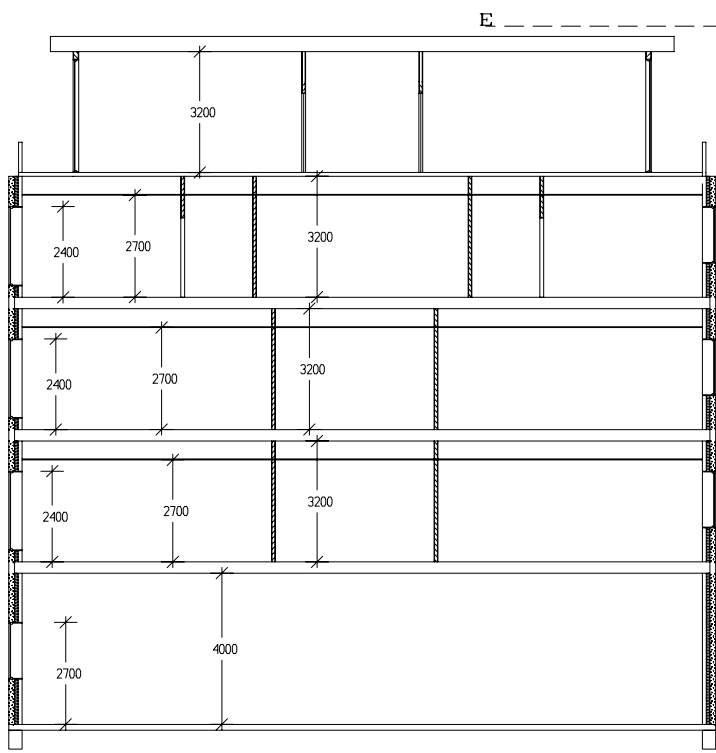
SNITT A-A
