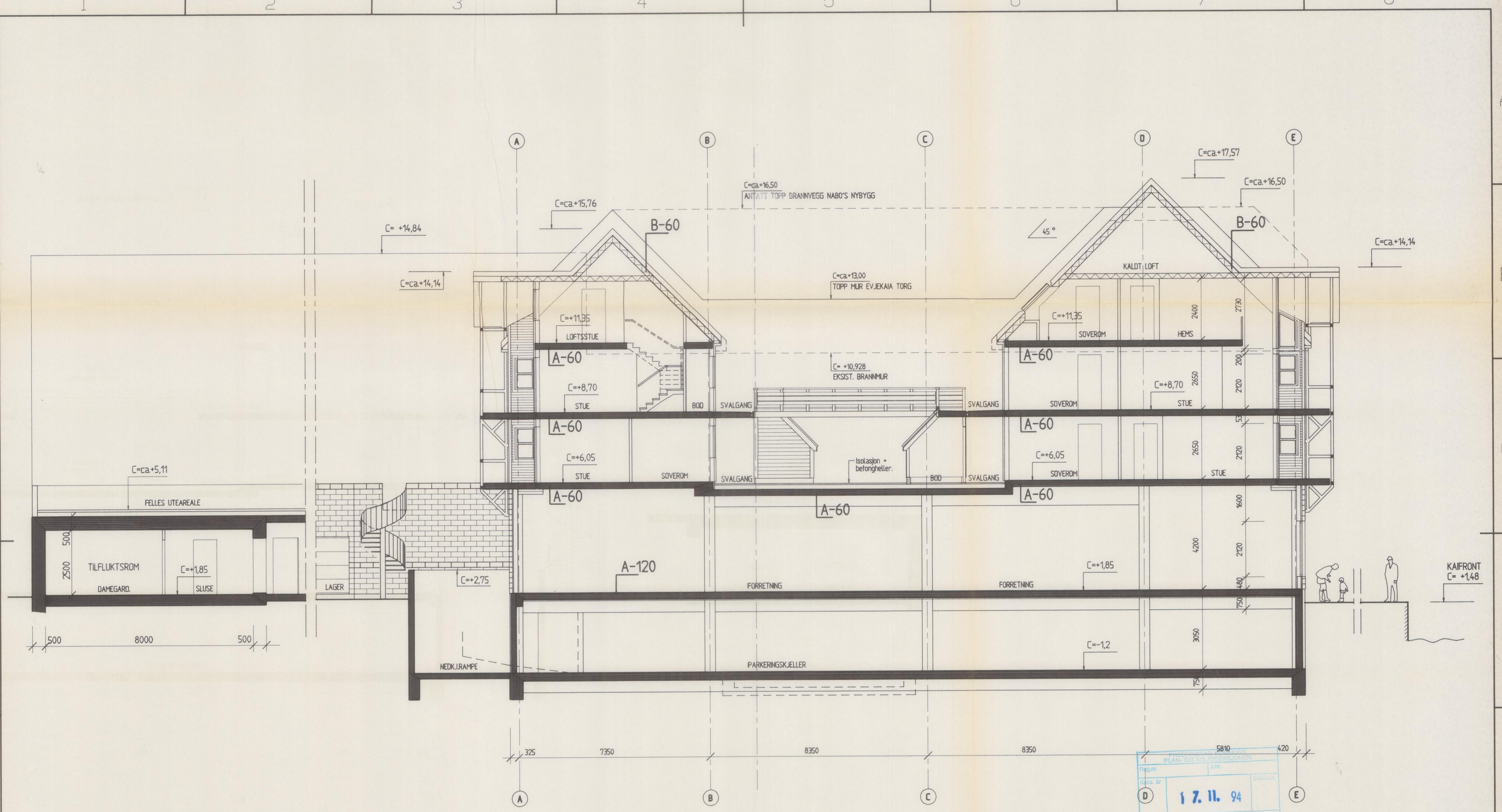
SNITT A-A
