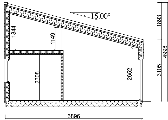
Snitt A-A
