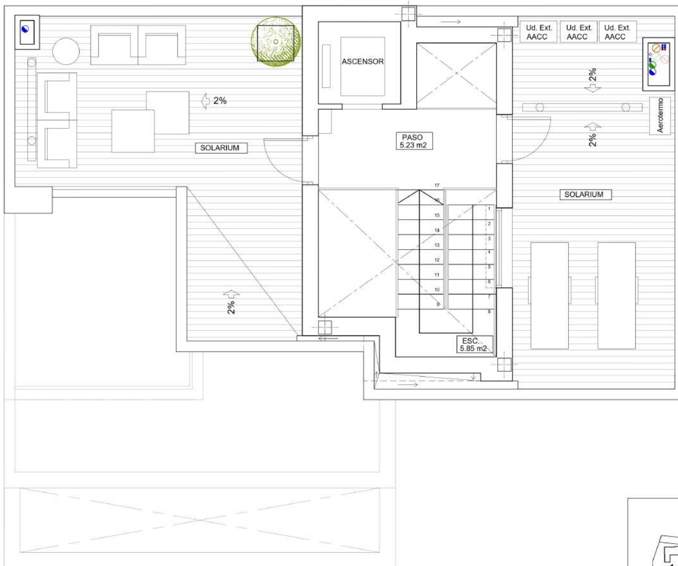
PLANTA SOLARIUM
