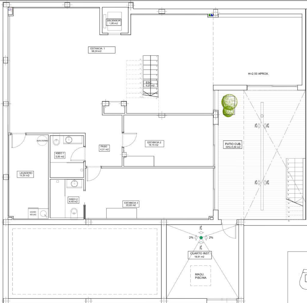
PLANTA SÓTANO. VIVIENDA 12
