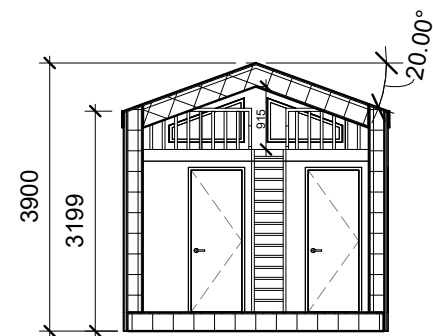
2 Snitt 1 : 100
