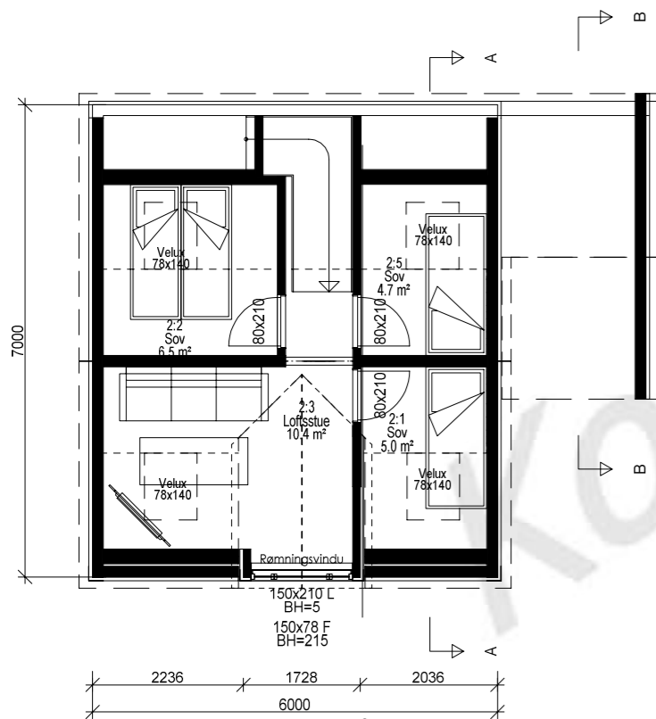
Loftsplan Bra=23,9m 2
