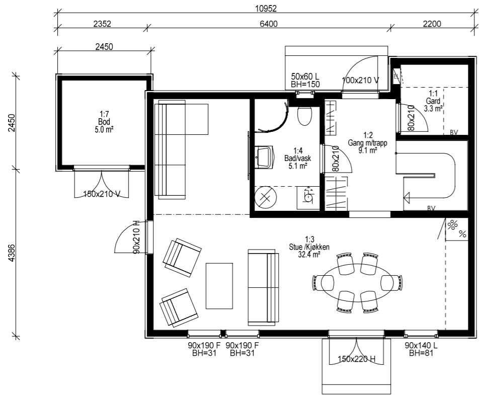
Plan 1. etasje. BYA=64,8m 2 / BRA=57,2m 2
