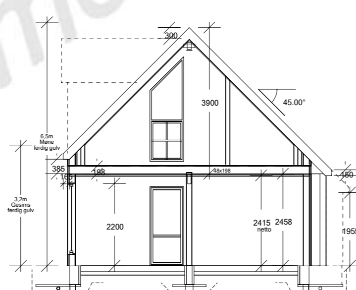
Snitt A-A
