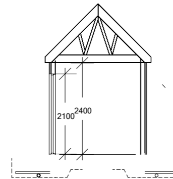
Snitt B-B
