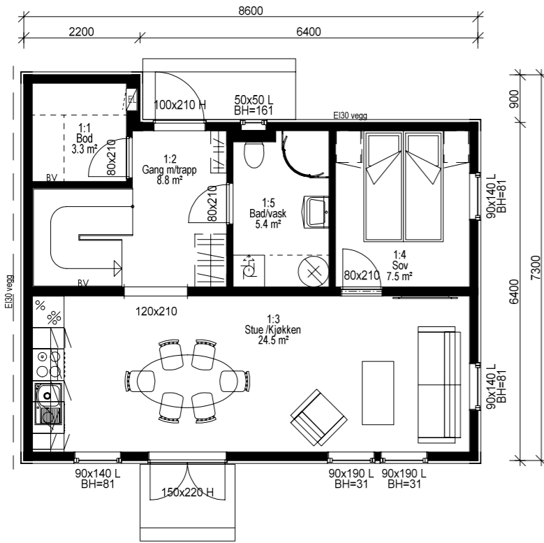
Plan 1. etasje. Brutto=58,7m 2 / Bra=51,9m 2
