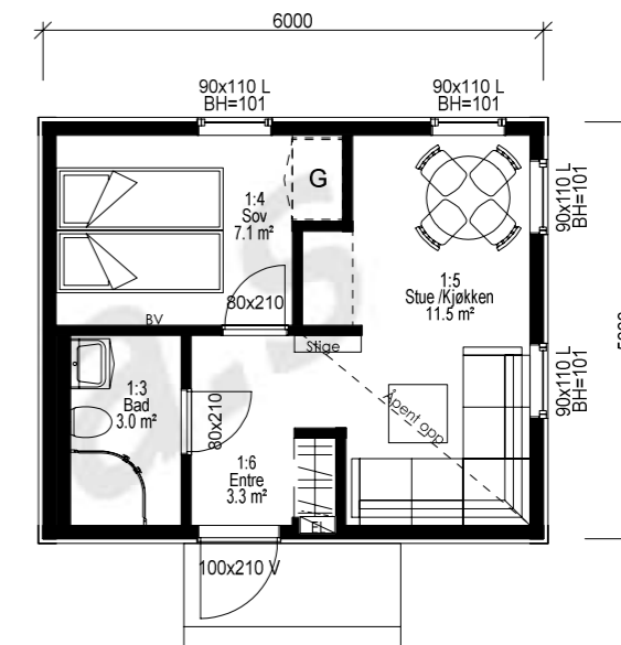
Plan 1.etasje. Brutto=31,2m 2 /Bra=26,6m 2
