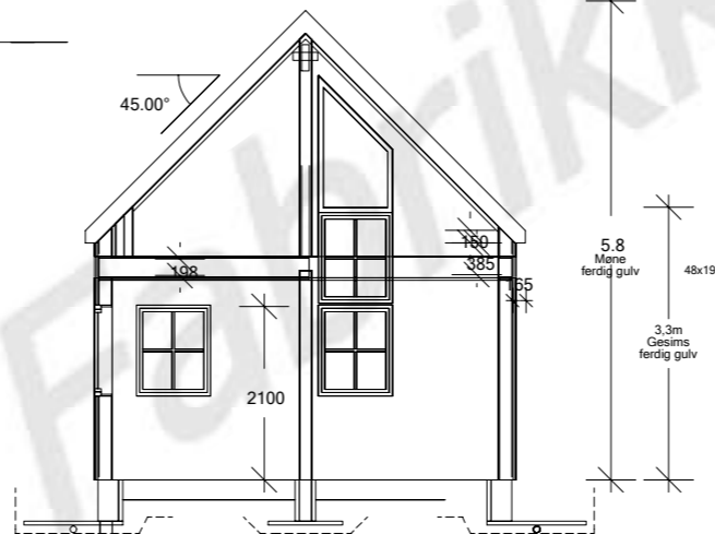
Snitt A-A
