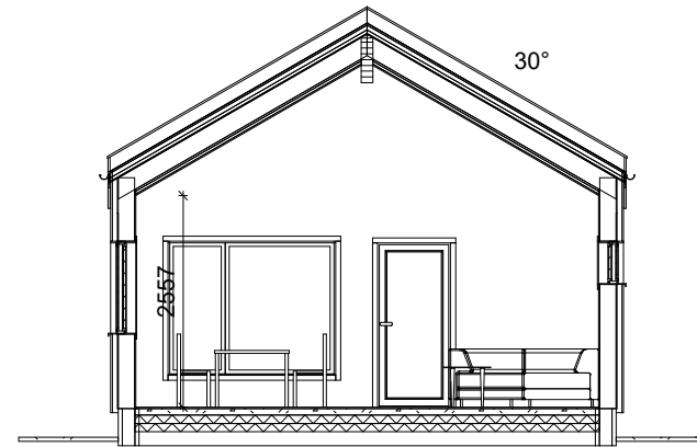
Snitt B-B
