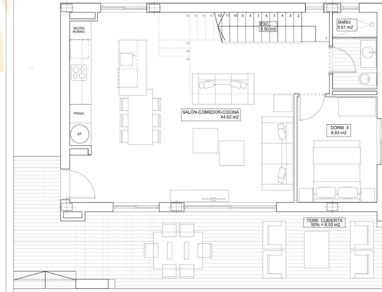
PLANTA BAJA. OPCIÓN SIN SÓTANO
