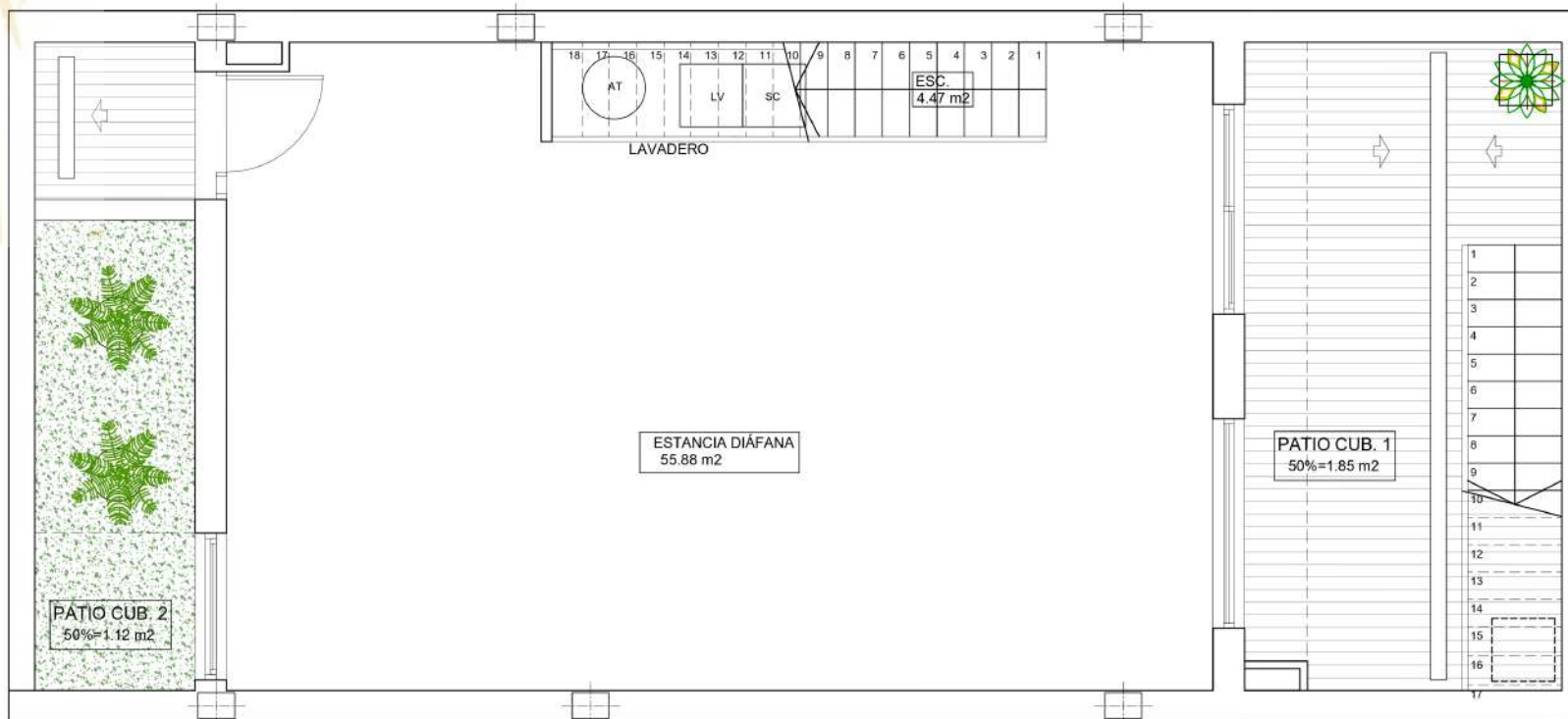
PLANTA SÓTANO
