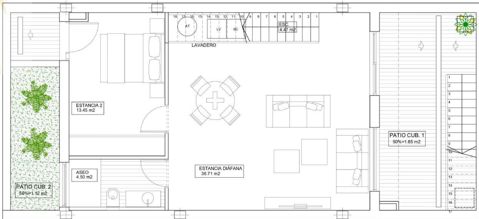
PLANTA SÓTANO
