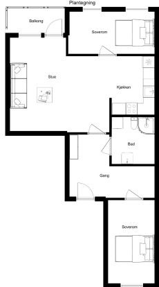
Plantegning av leiligheten.
