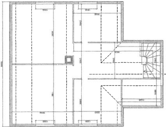
LOFTSPLAN 59,7 M2 (MÅLBART AREAL)
