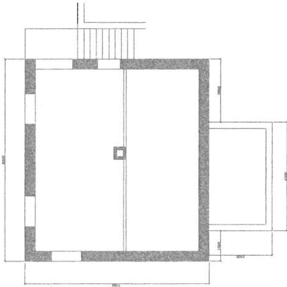
KJELLARPLAN 46,6 M2
