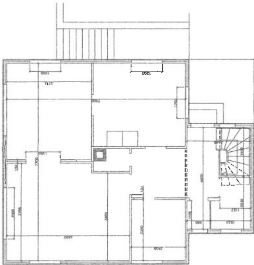
HOVEDPLAN 63,8 M2
