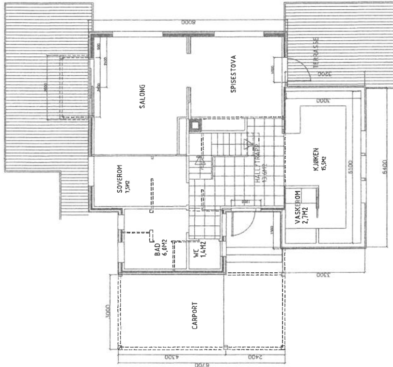
HOVEDPLAN 18,6 M2 TILBYGG
