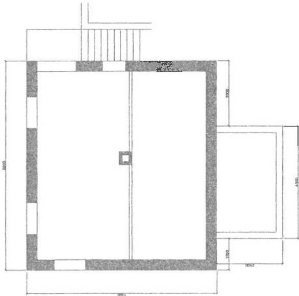
KJELLARPLAN 46,6 M2
