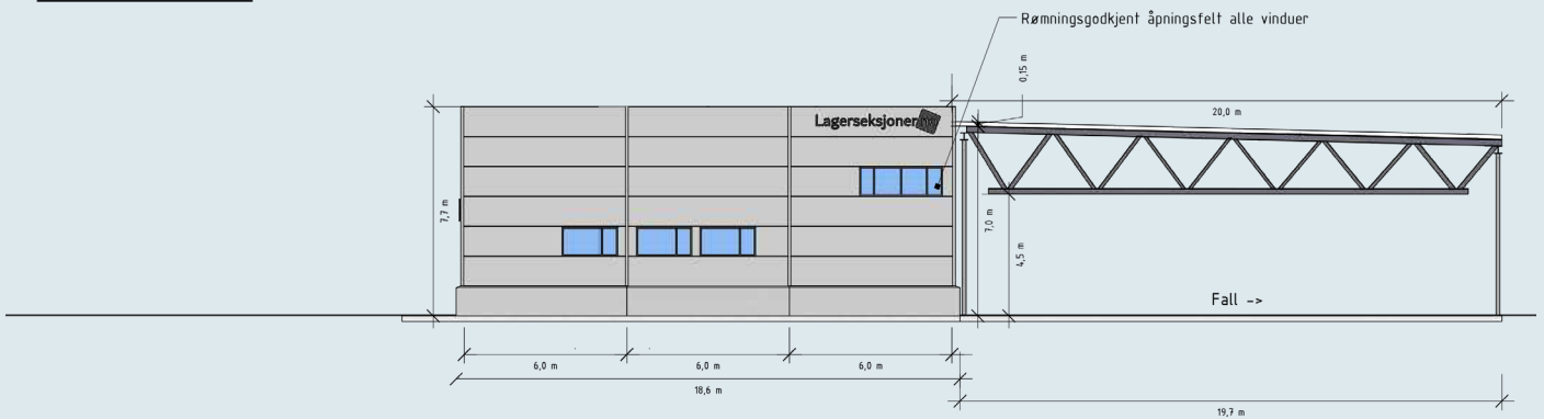
Fasade Sør
