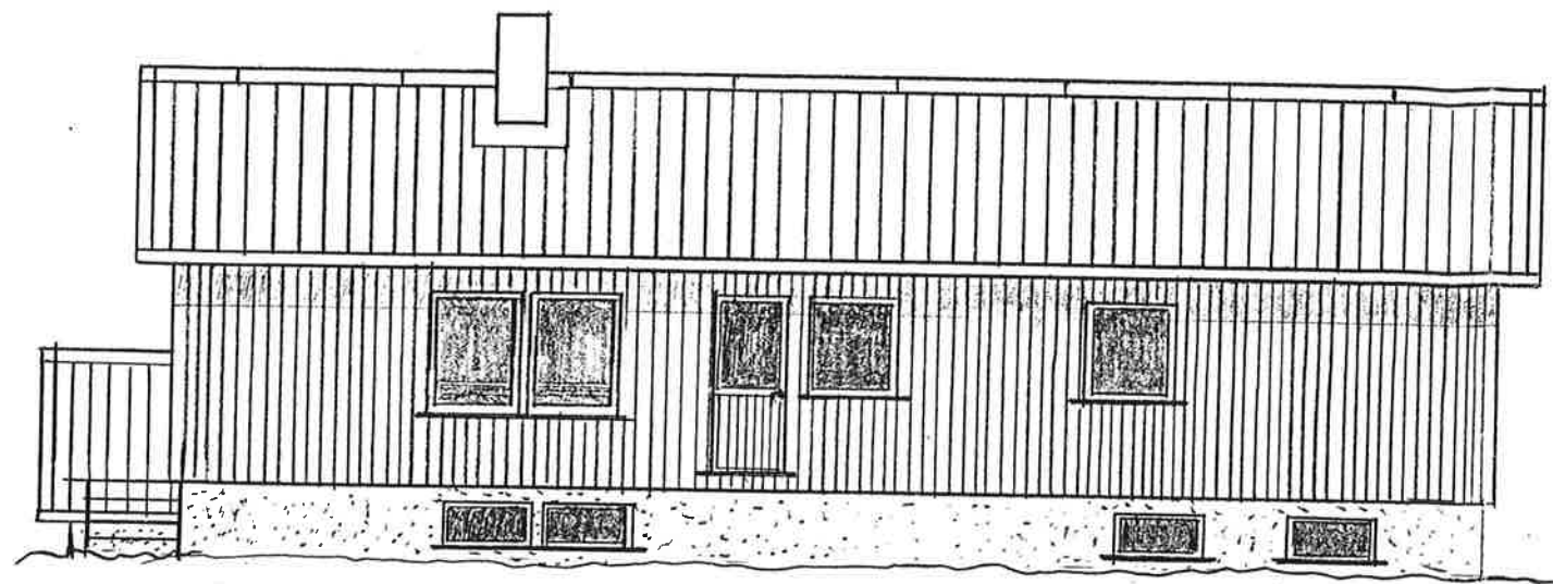
FASADE ØST
