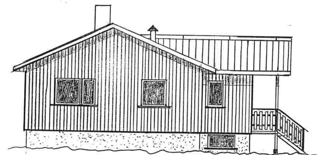
FASADE NORD
