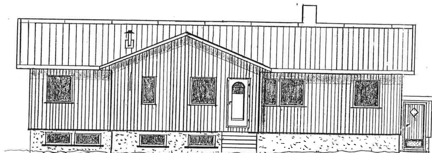
FASADE VEST
