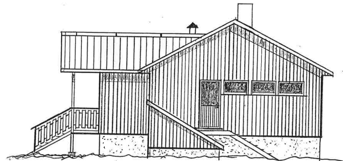
FASADE SØR
