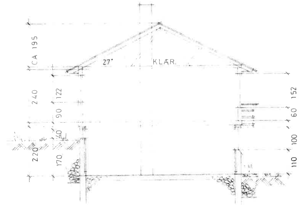
TVERRSNITT.
