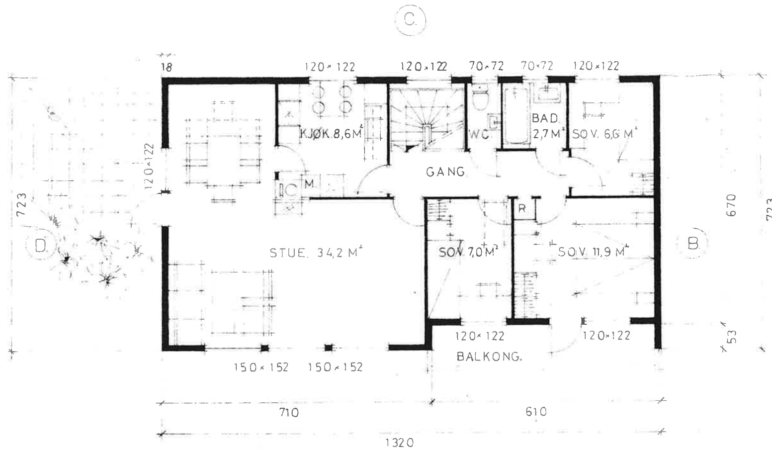
PLAN 1 ETASJE.
