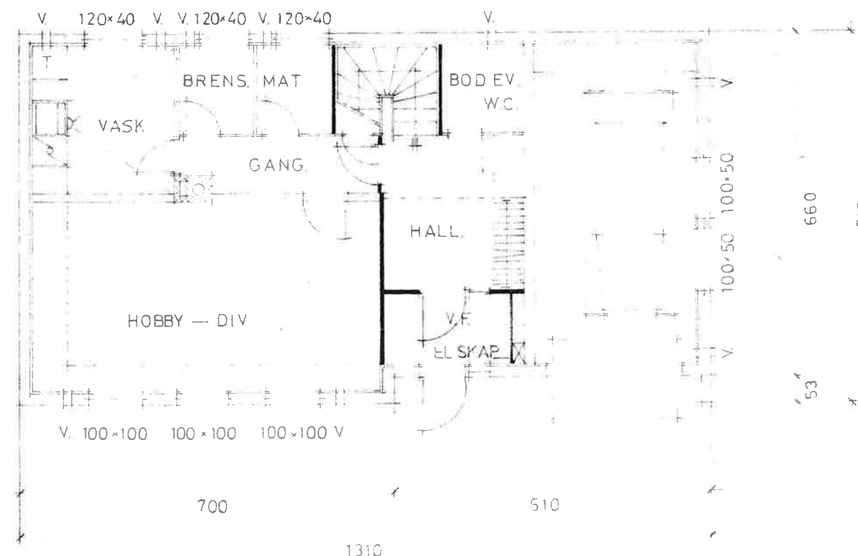
PLAN KJELLER.
