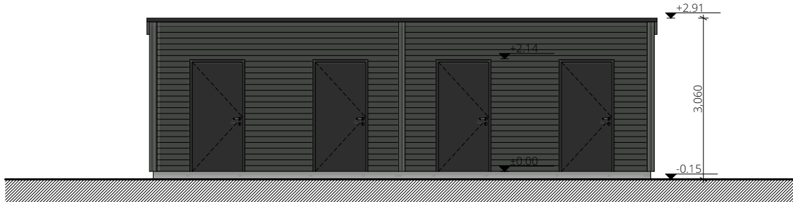
FASADE C
