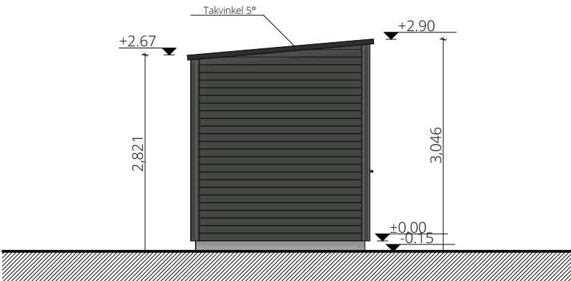
FASADE D
