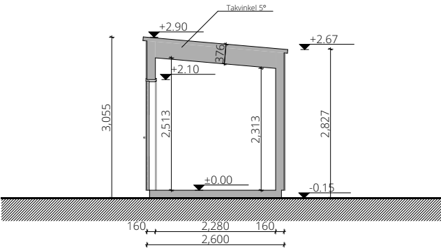
SNITT A-A
