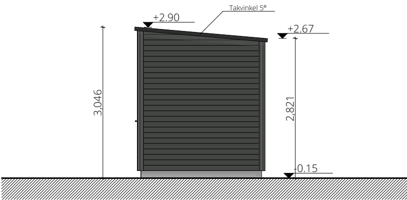
FASADE B
