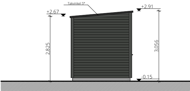
FASADE D
