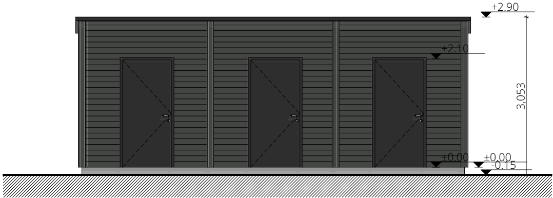
FASADE C
