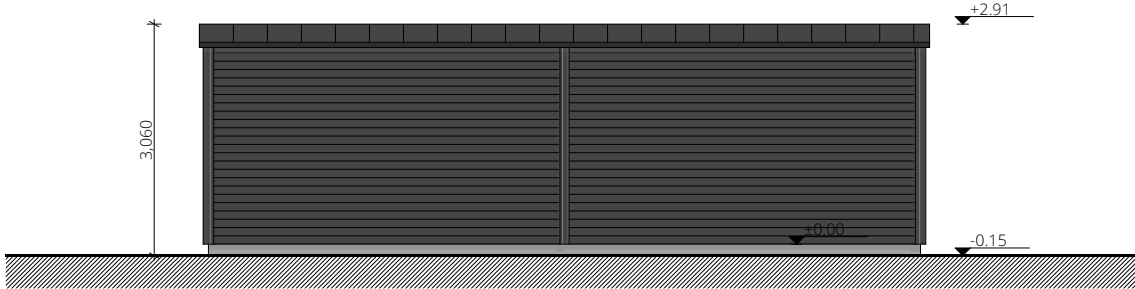
FASADE A
