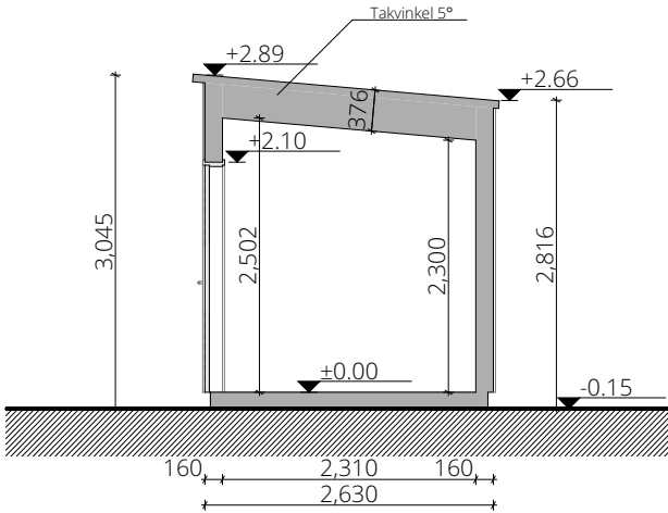
SNITT A-A
