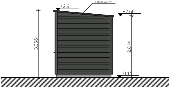
FASADE B
