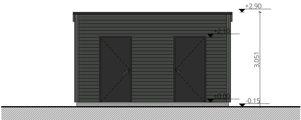
FASADE C
