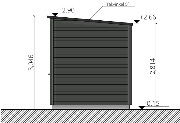
FASADE B
