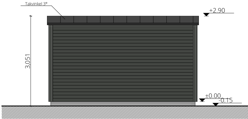
FASADE A
