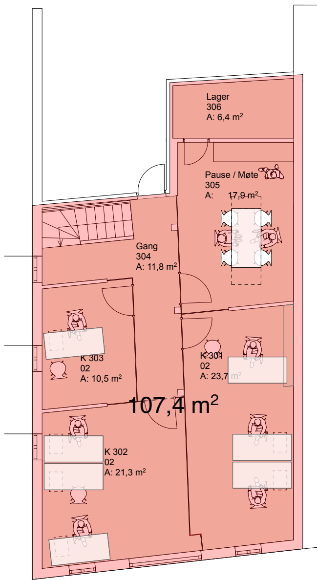
3 etasje
