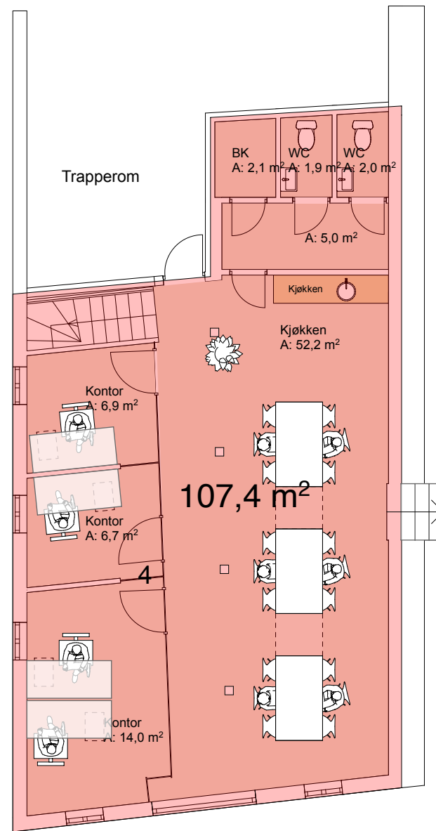
2 etasje
