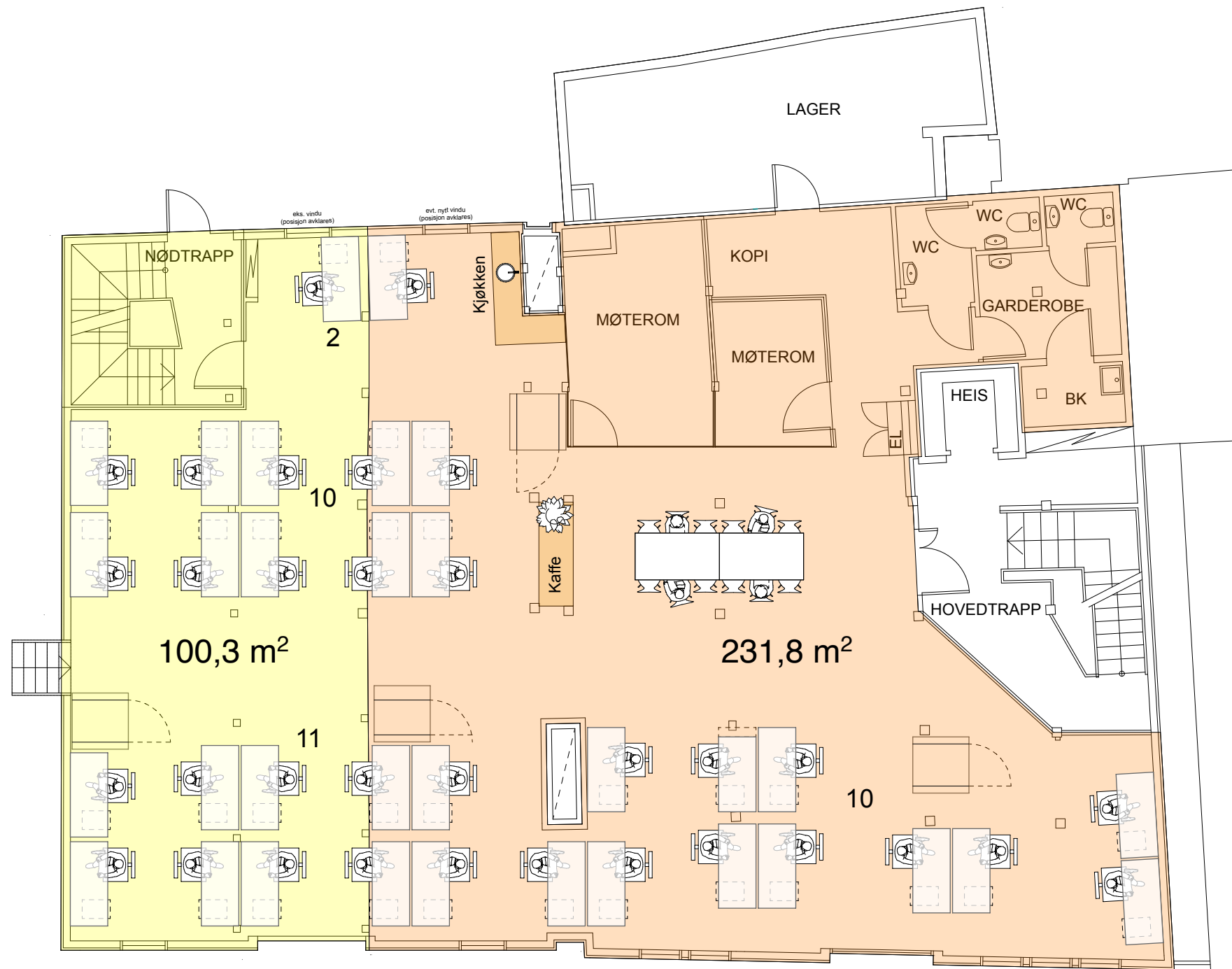
2 etasje
