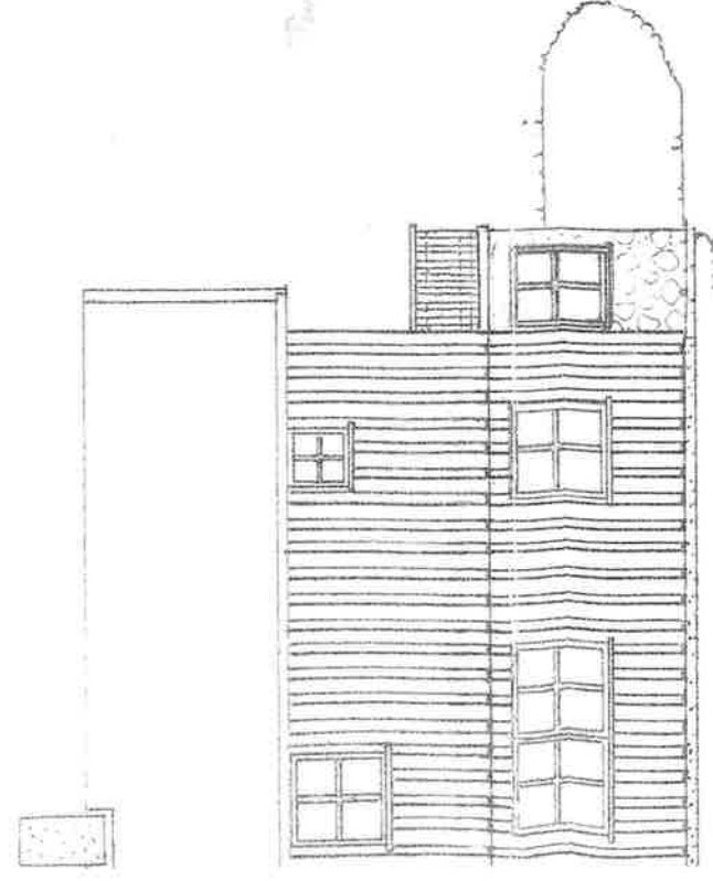
MOT SØR
