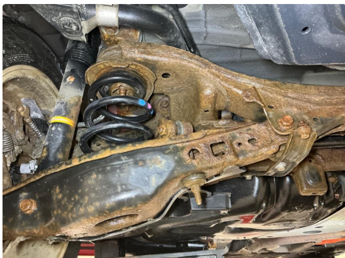
1.2 Korrosjon undervogn
