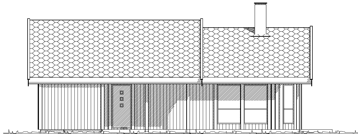
FASADE NORD
