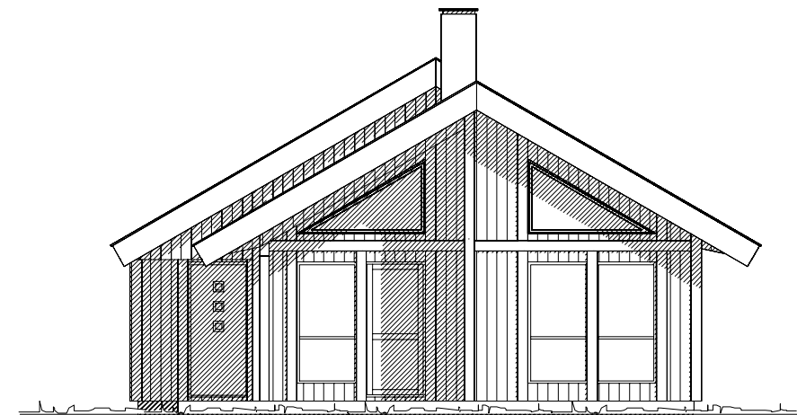
FASADE VEST
