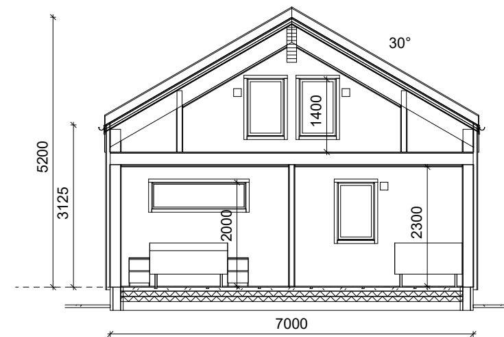
SNITT A-A
