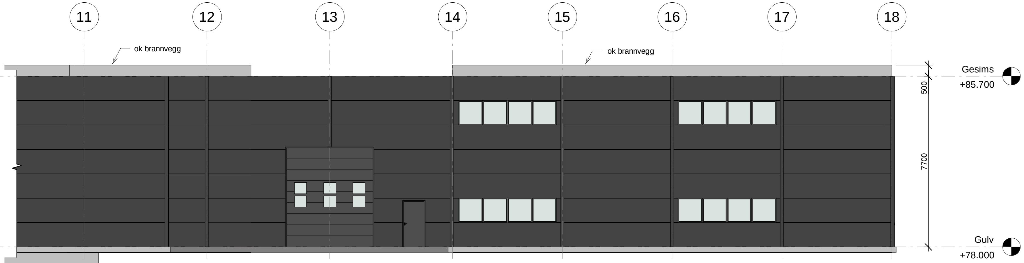
Stemmane 28 - Sør 1 : 100
