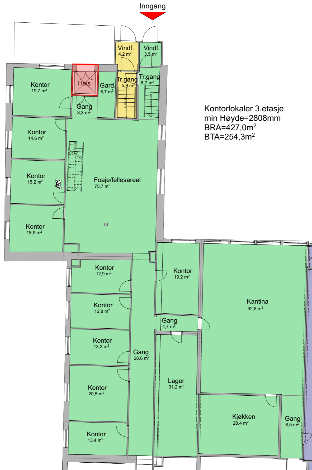
Plan 1:150
