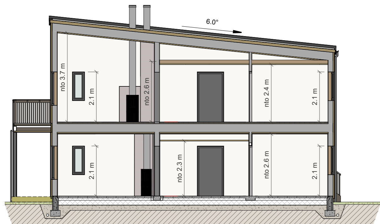
Snitt A1
