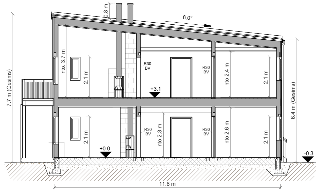
Snitt A-A
