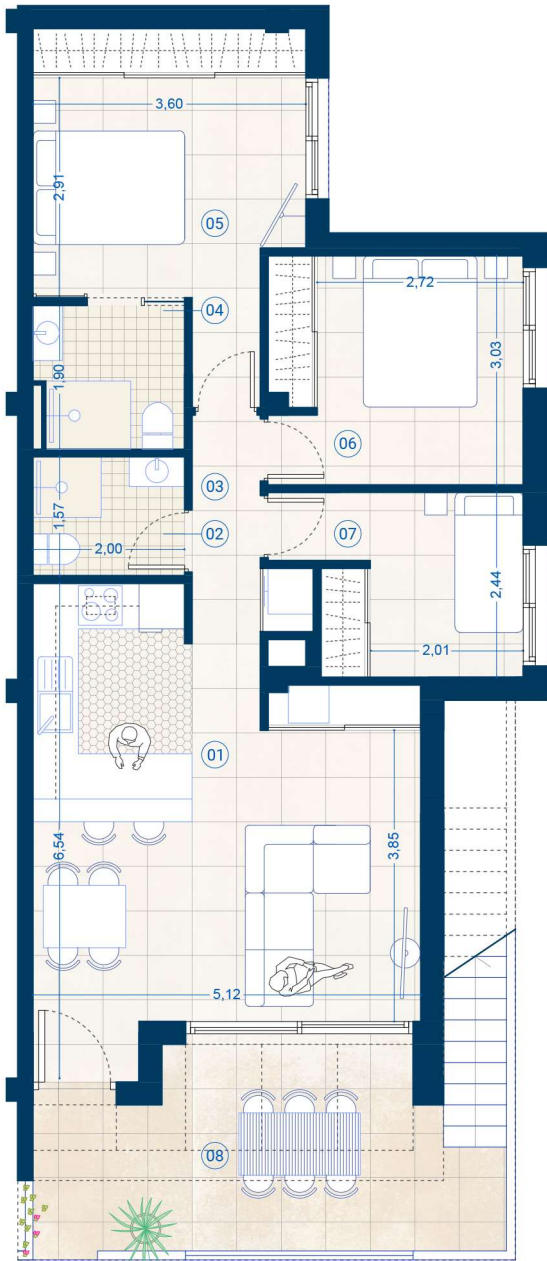
VIVIENDA EN PLANTA PRIMERA/HOUSE IN FIRST FLOOR
