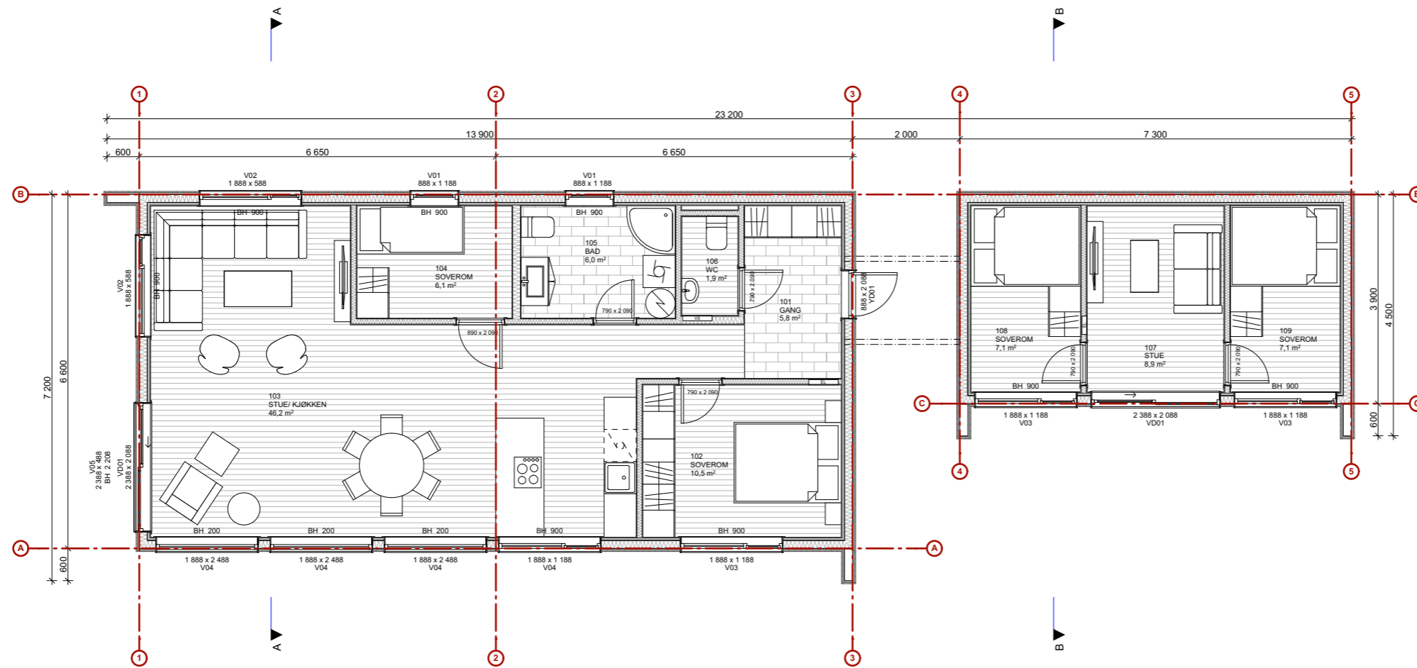
1:100 1. Etasje
