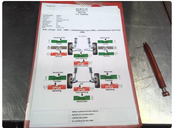
2.1 4-hjulsmåling/forstillingskontroll. Må justeres
