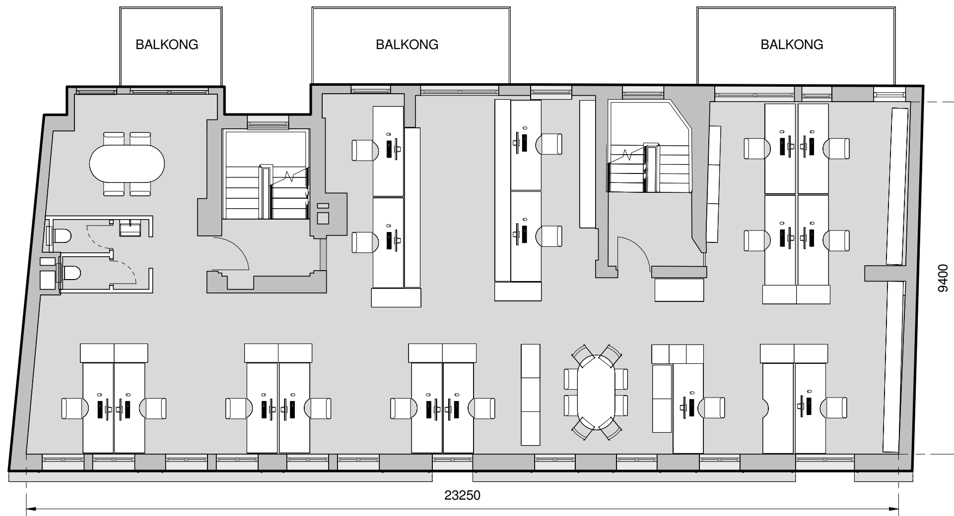
1 Plan 04 1 : 100
