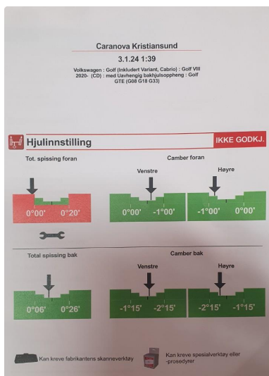
2.1 4-hjulsmåling/forstillingskontroll
